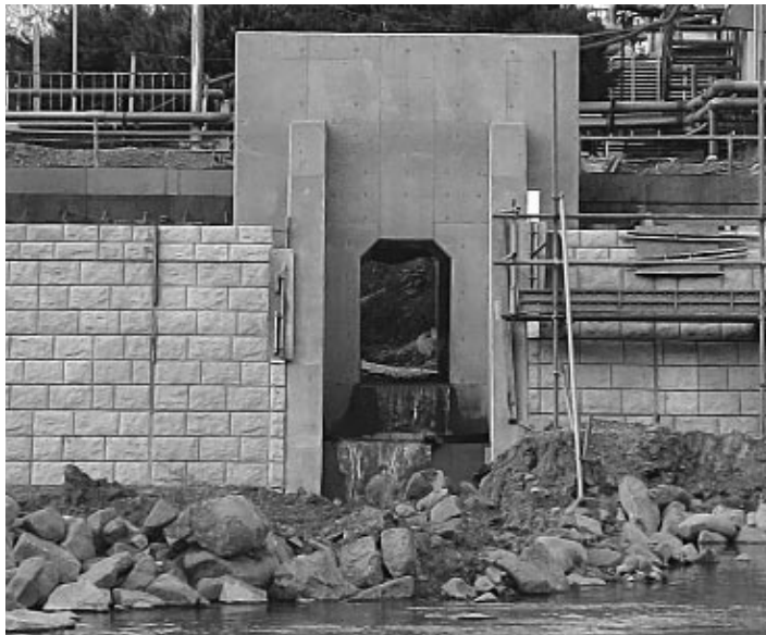
△ 大雨時の気仙川と沢水の氾濫防止に設置されるフラップゲート (世田米和山)
